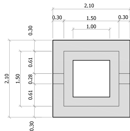
DEFINICIÓ GEOMÈTRICA. PLANTA
