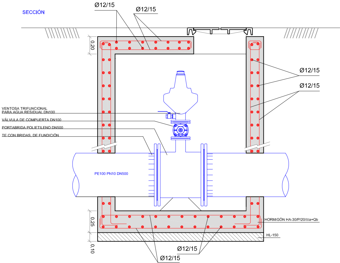
ARQUETA PARA VENTOSA. EMISARIO
