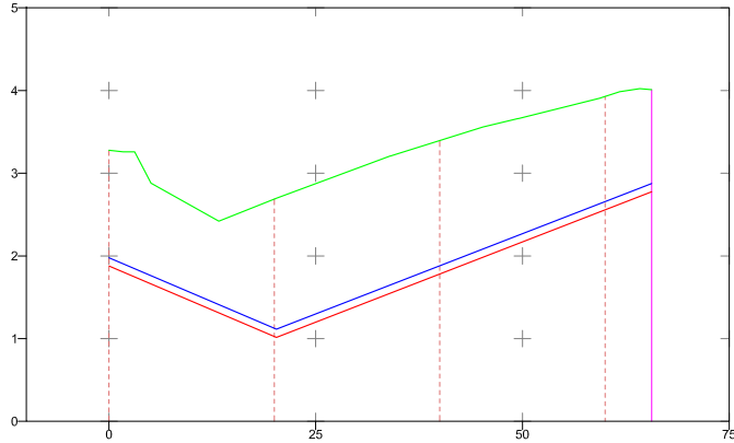
IMPULSIÓN CLUB DE VELA. PK 0+000.000 - PK 0+065.628
