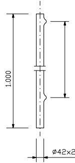
PIE DE BARANDILLA
