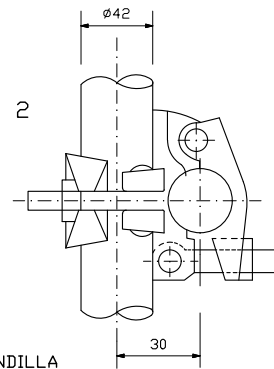
ABRAZADERA DOBLE FIJA DE HIERRO FORJADO
