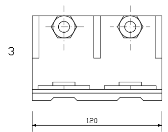
ABRAZADERA DE EMPALME
