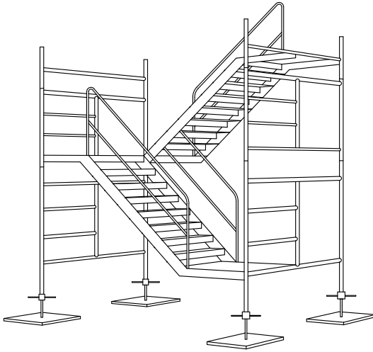
ESCALERA INTERIOR
