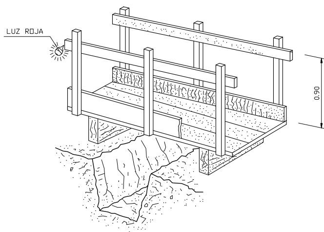
DETALLE DE PASARELA PEATONES
