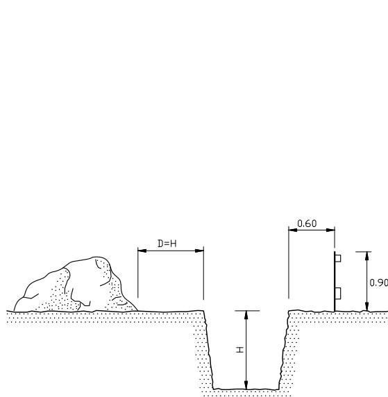
PROTECCION DE ZANJAS EN TERRENO ARENOSO
