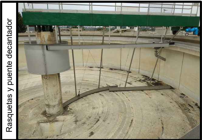
Puente decantador y pivote central
