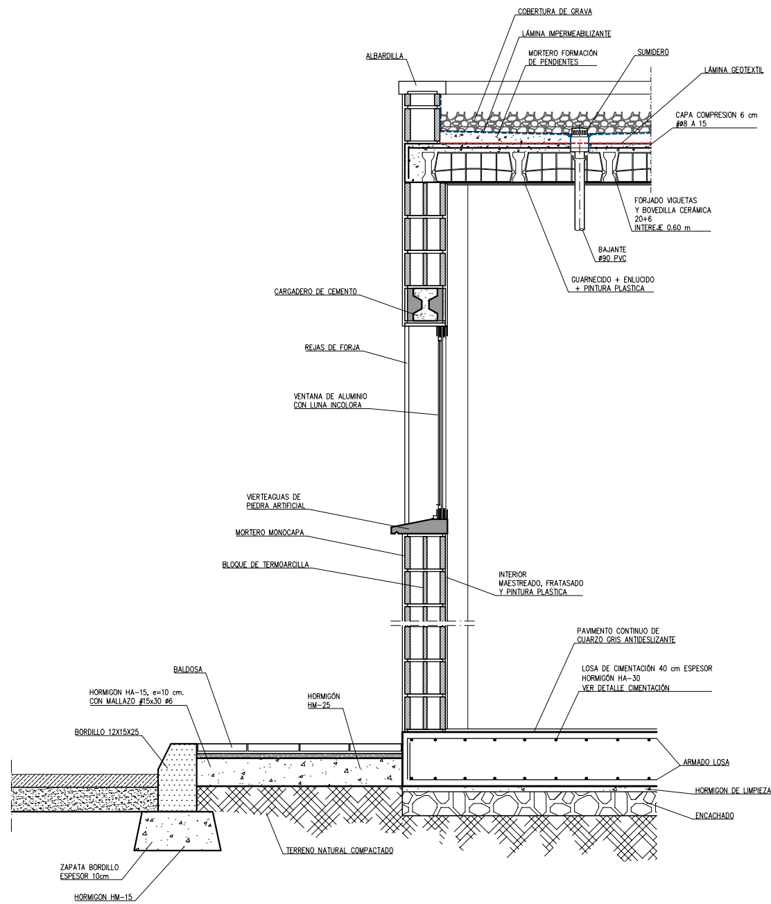
DETALLE CONSTRUCTIVO
