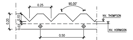
DETALLE VERTEDERO
