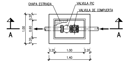
PLANTA ESCALA: 1/75
