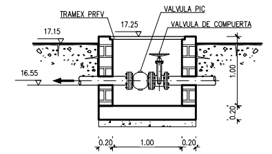
SECCION A-A ESCALA: 1/75
